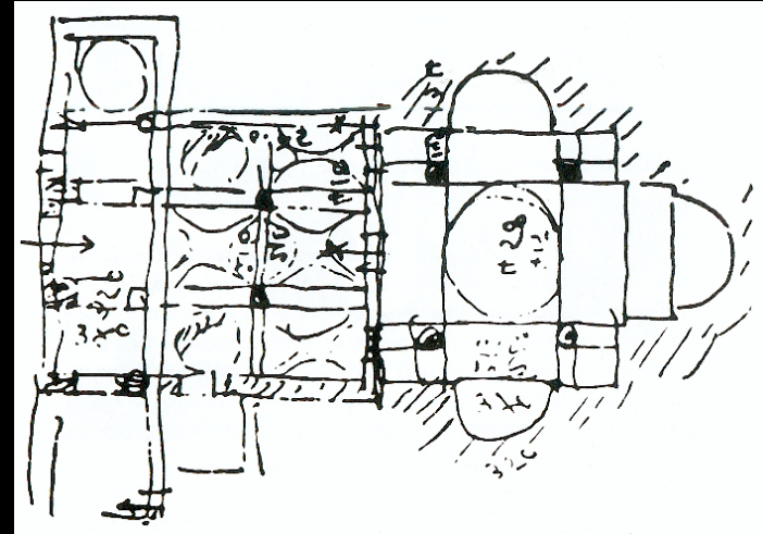
Η εκκλησία της μονής Φιλοθέου με διάφορες σημειώσεις
