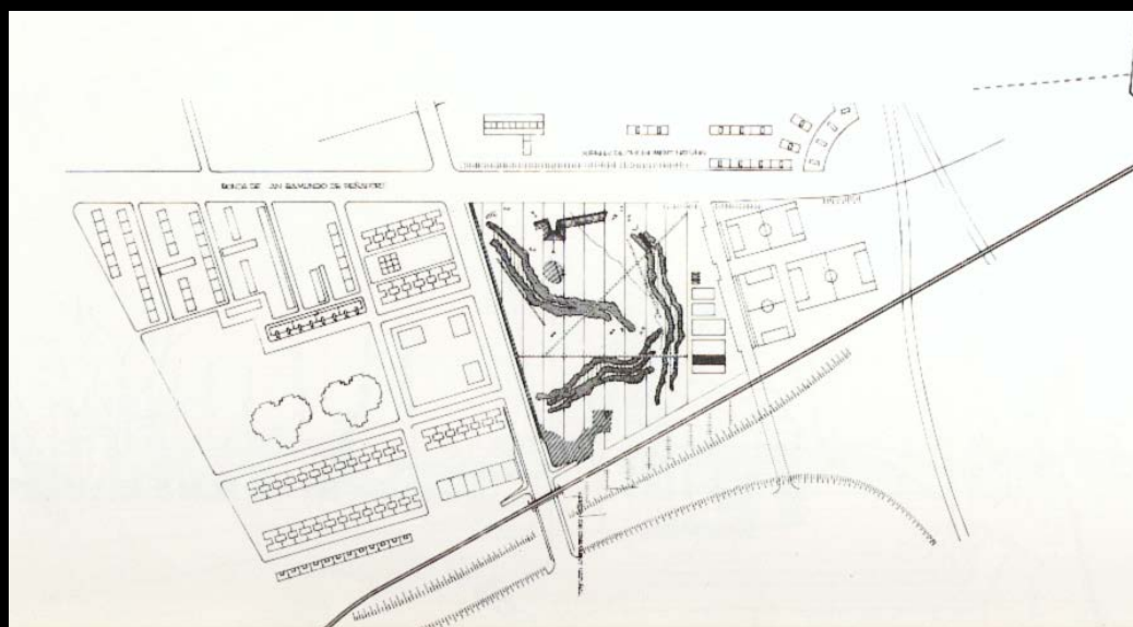
Σχέδιο για το Πάρκο del Besos, Βαρκελώνη, 1982
